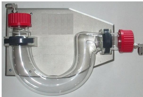
Abb. 1: APSON Glas-Siphon GSI-1019
