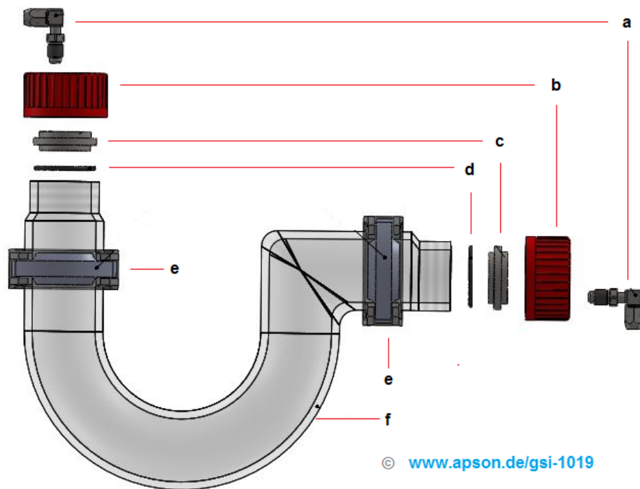
Abb. 2: APSON Glas-Siphon GSI-1019 - Aufbau
