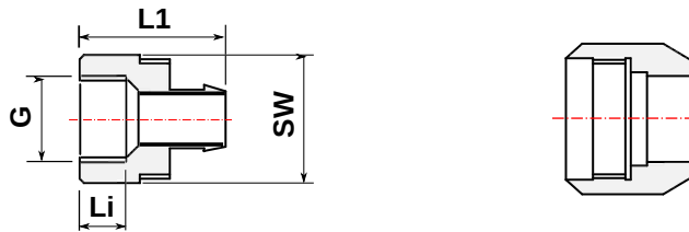
APSON SL-Gerade-Verschraubungen G1/4" mit Innengewinde x 90° Konusdichtung - Maßangaben
